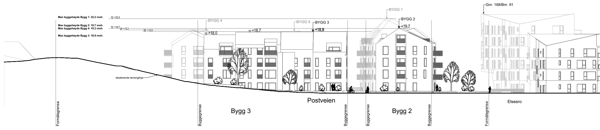
7 Snitt 1:500
