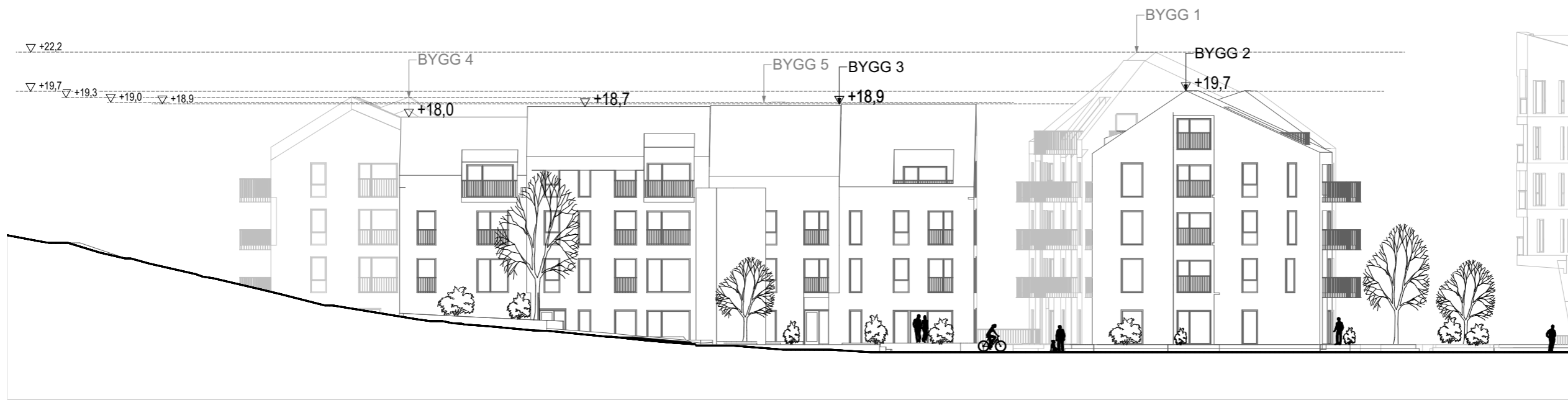
7 Snitt 1:300
