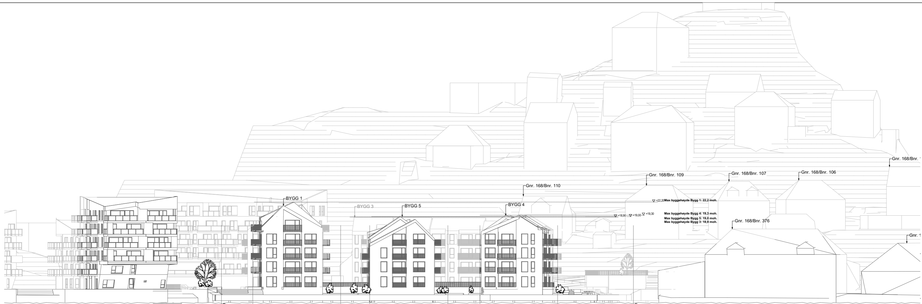
5 Snitt 1:500 ELSESRO HOP Formålsgrænse Flytebrygge Byggegrænse Bygg 1 Byggegrænse BYGG 3 BYGG 5 BYGG 4 Byggegrænse Byggegrænse Kaifront Bygg 5 SANDVIKSODER 78 Byggegrænse Byggegrænse Bygg 4 Byggegrænse KATTAHOPEN Formålsgrænse HOLMEFJORBODEN Gnr. 168/Bnr. 109 Gnr. 168/Bnr. 107 Gnr. 168/Bnr. 106 Gnr. 168/Bnr. 110 Gnr. 168/Bnr. 376 Gnr. 1 Max byggeheide Bygg 1: 22,2 moh. Max byggeheide Bygg 4: 19,3 moh. Max byggeheide Bygg 5: 19,0 moh. Max byggeheide Bygg 3: 18,8 moh. ▽ +22,20 ▽ +18,90 ▽ +19,00 ▽ +19,30
