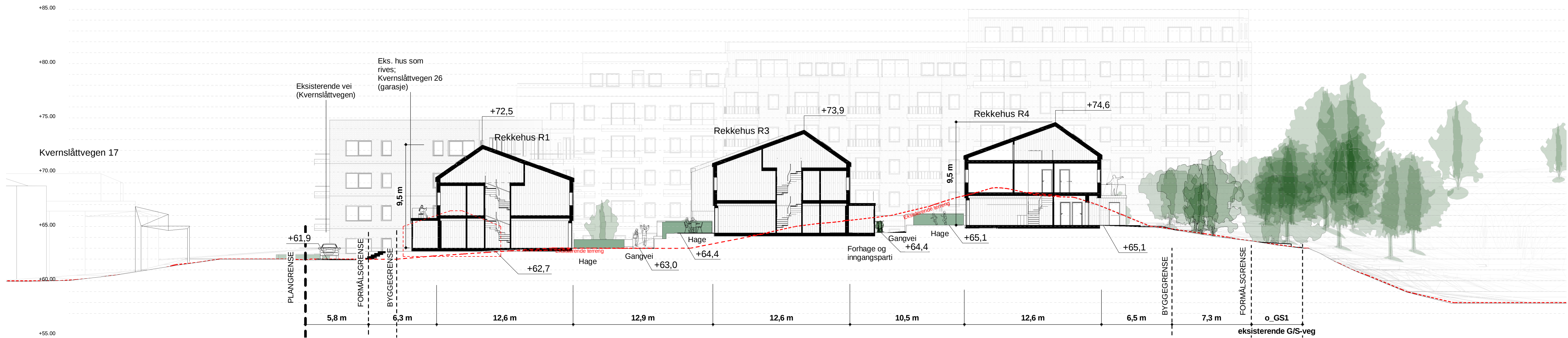
Snitt E - rekkehus 1 : 200
