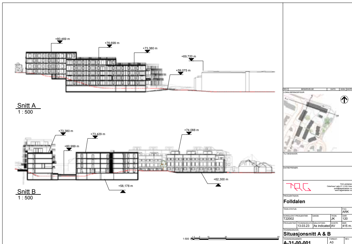
Situasjonsplan Folldalen – snitt. Kjelde: Sweco Architects AS.
