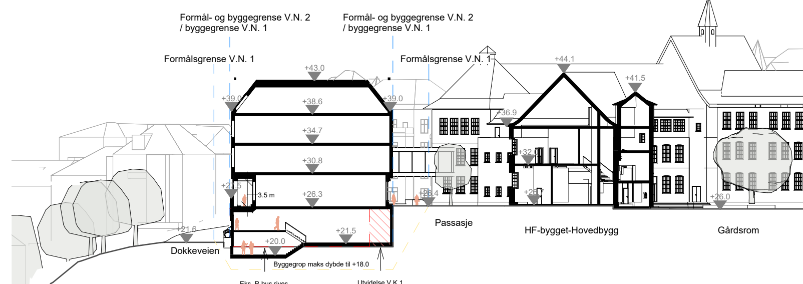
Snitt CC 1 : 500
