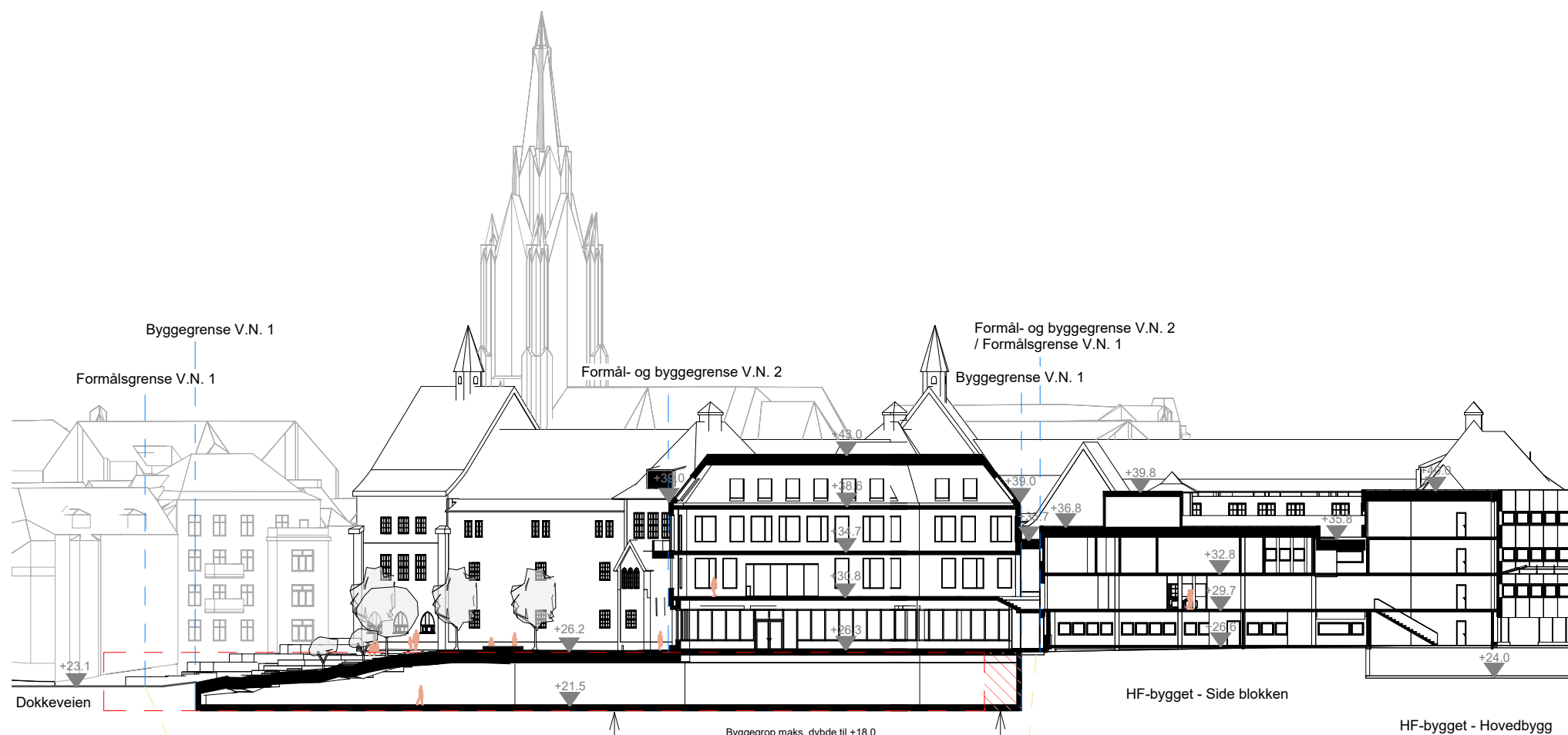
Snitt AA 1 : 500
