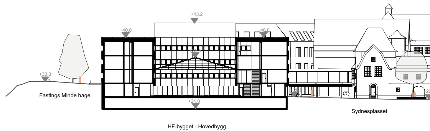
Snitt FF 1 : 500
