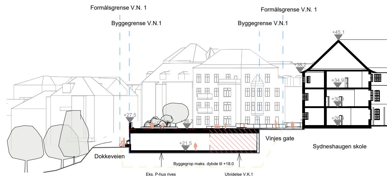
Snitt BB 1 : 500
