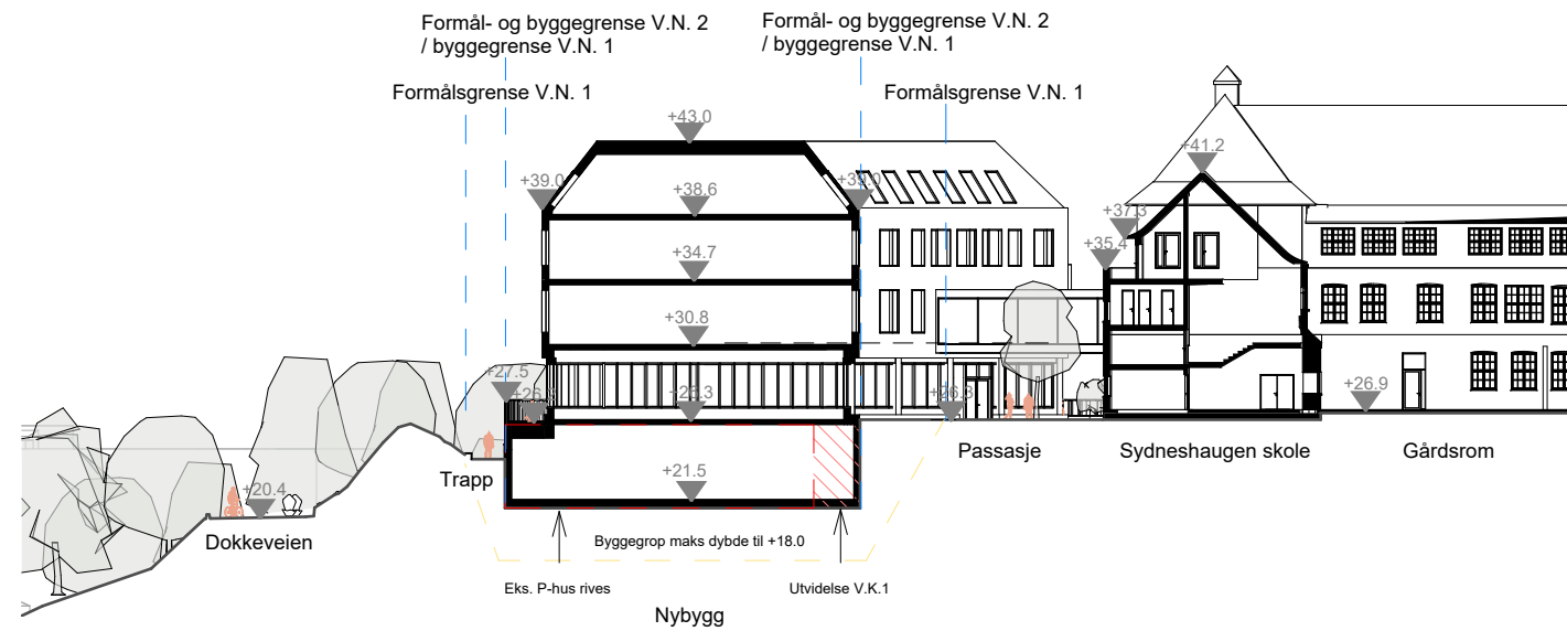
Snitt DD 1 : 500
