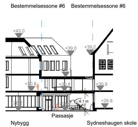
Snitt GG 1 : 500
