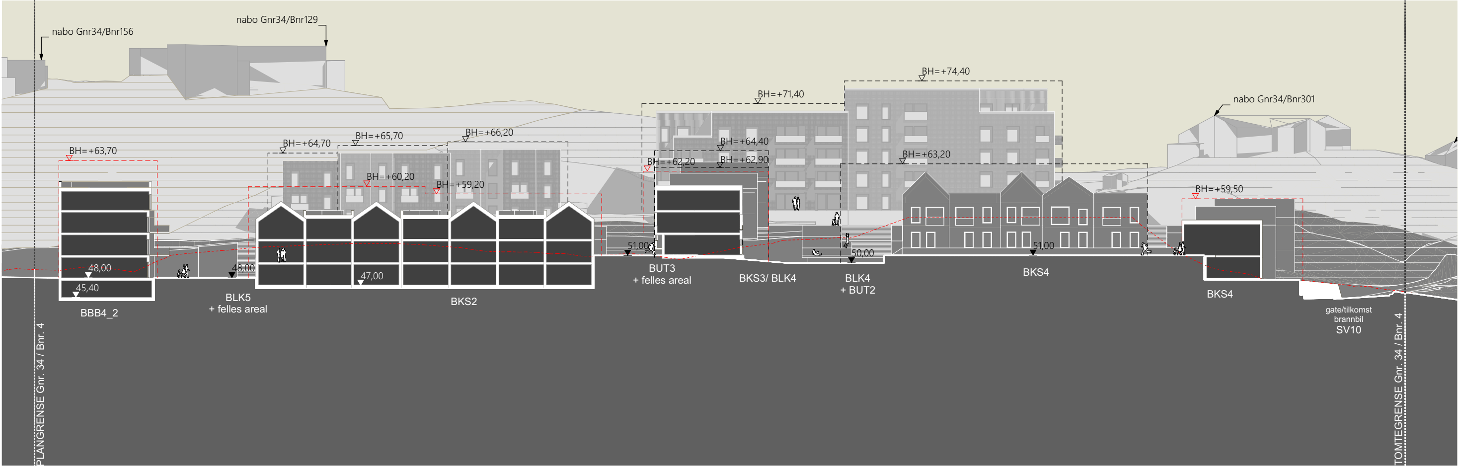
Terrengsnitt D-D
