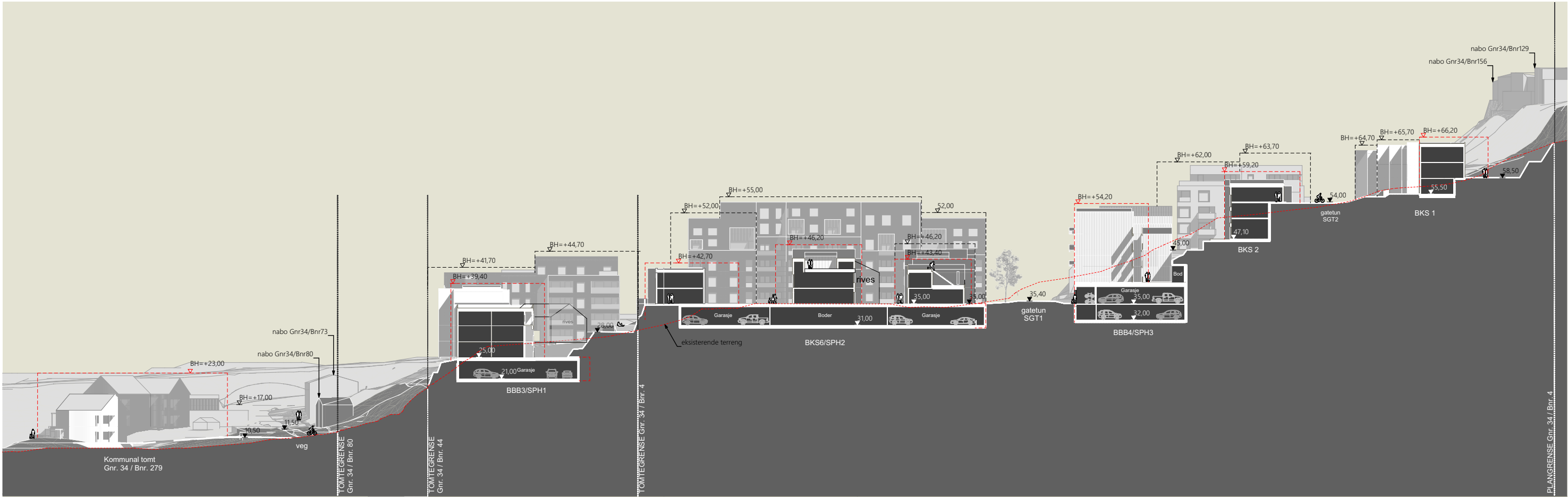
Terrengsnitt A-A
