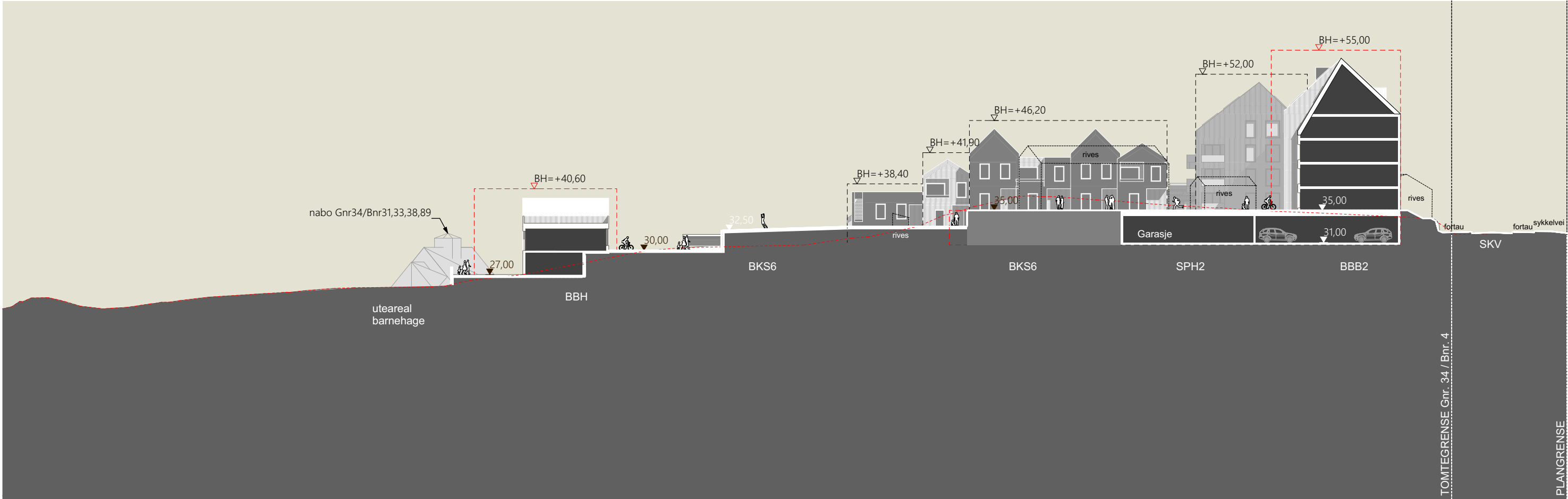
Terrengsnitt C-C
