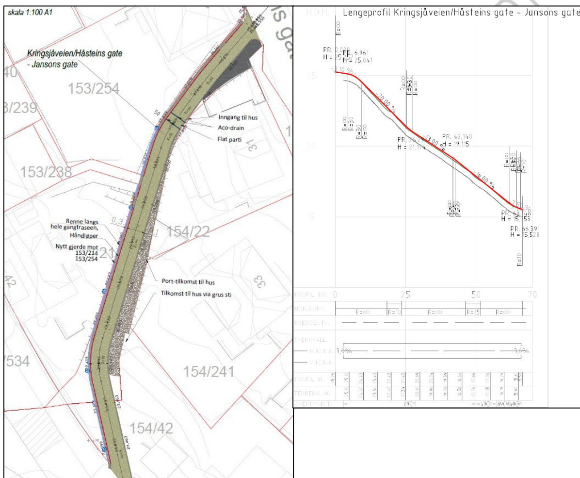
Figur 36. Detaljtegning i plan og lengdeprofil av o_GG Kringsjåveien/Håsteinsgate – Jansons gate.
