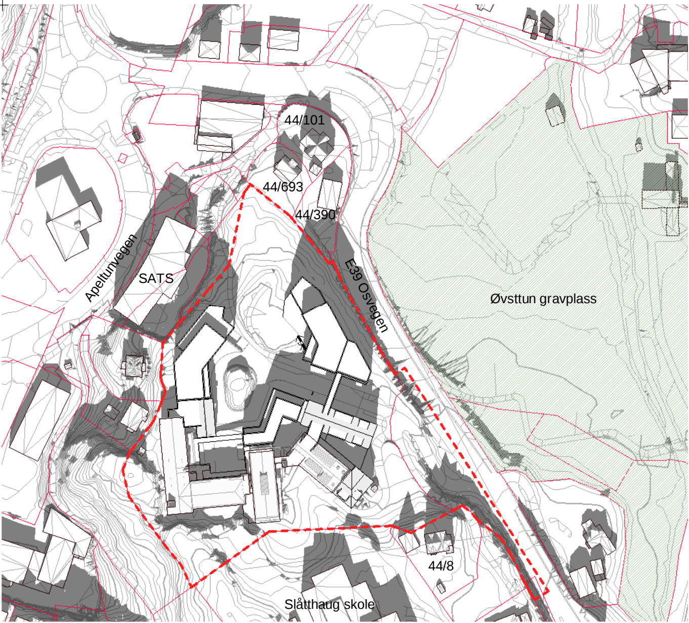
01D - 21. mars kl. 13 1 : 2000
