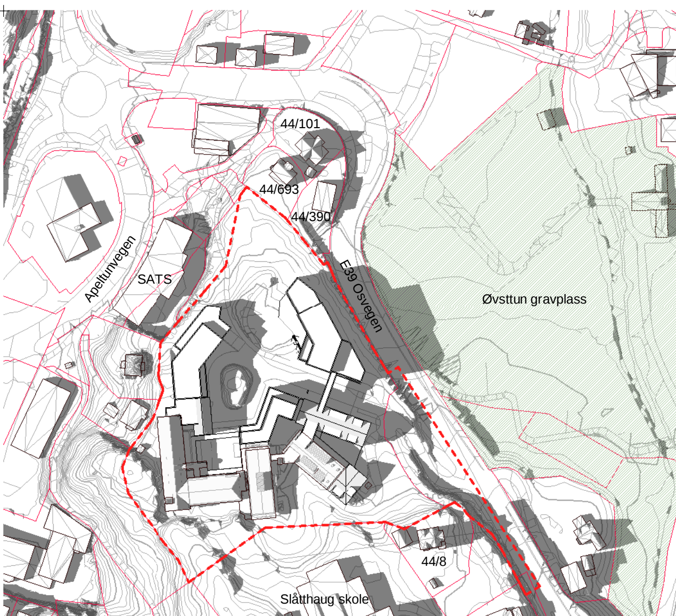
09D - 20. mai kl. 18 1 : 2000
