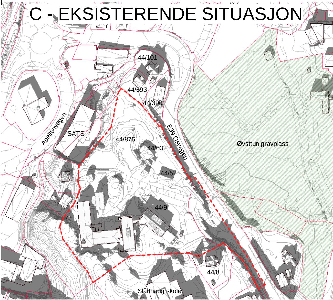
02C - 21. mars kl. 14 1 : 2000
