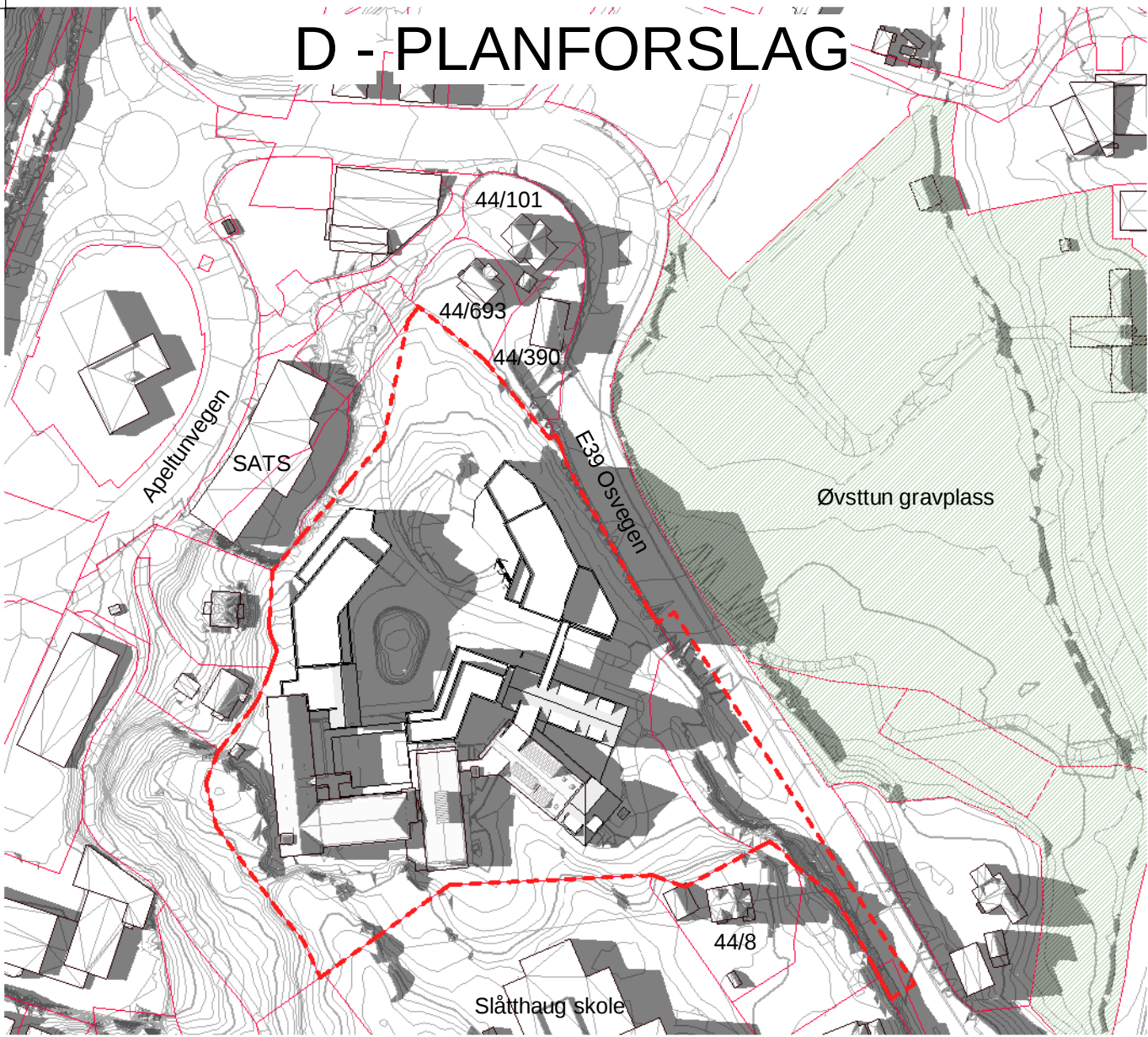
14D - 21. juni kl. 19 1 : 2000
