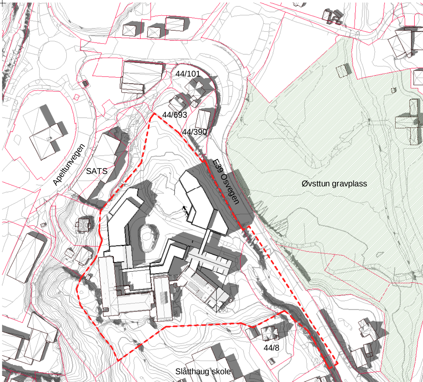
12D - 21. juni kl. 17 1 : 2000
