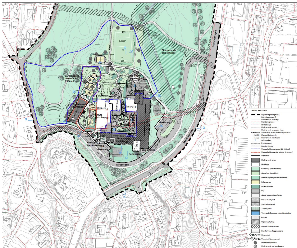
Figur 5.3.1.2 – Utsnitt av illustrasjonsplan datert 26.08.2025 viser mulig organisering av utearealene til skolen og barnehagen
