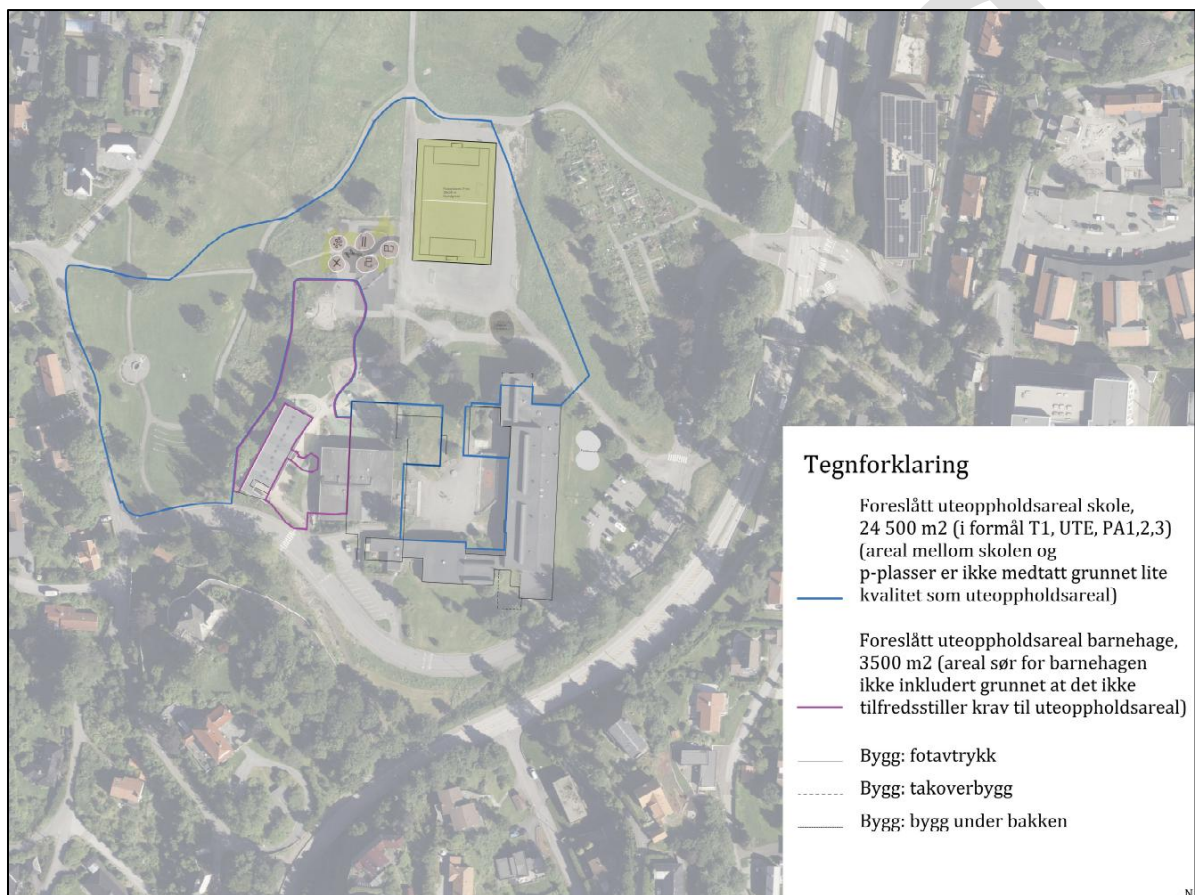
Figur 5.3.1.1. – Utearealer for hhv. Storetveit skole (blått omriss) og Storetveit barnehage (lilla/blå omriss)
