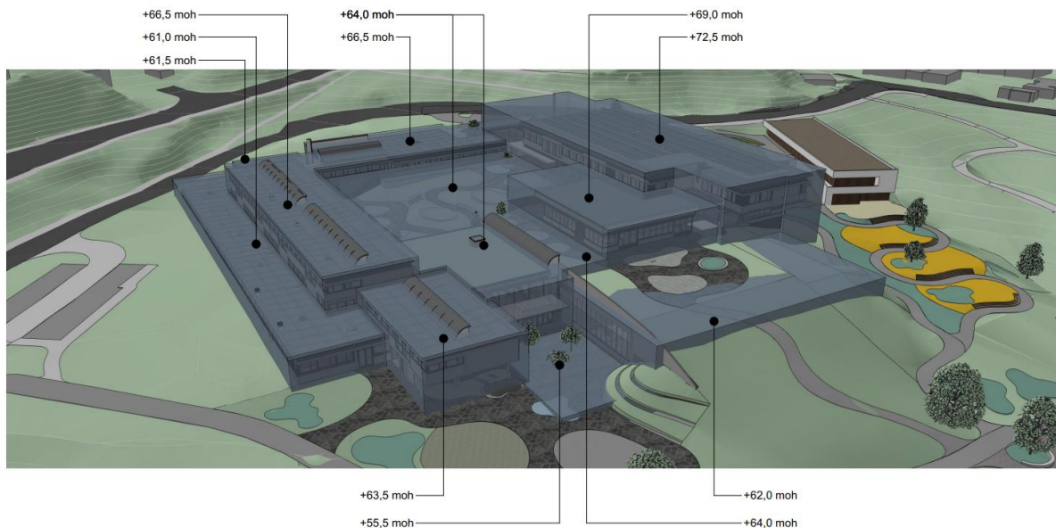
Figur 5.2.1.1 – Illustrasjon som viser foreslått maksimal byggehøyde (blått volum), sett i forhold til forprosjektert bygg per juni 2025
