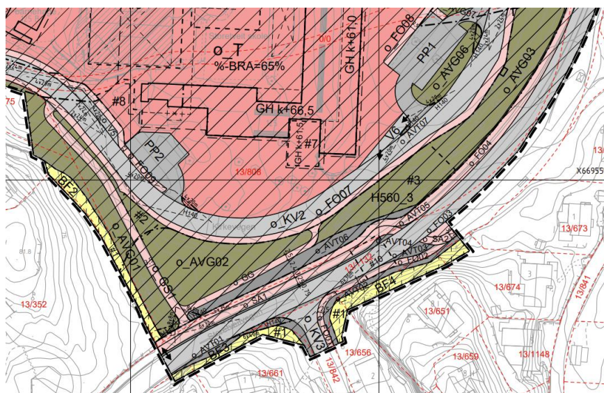
Figur 24 Sykkelveg med fortau langs Storetveitveien
