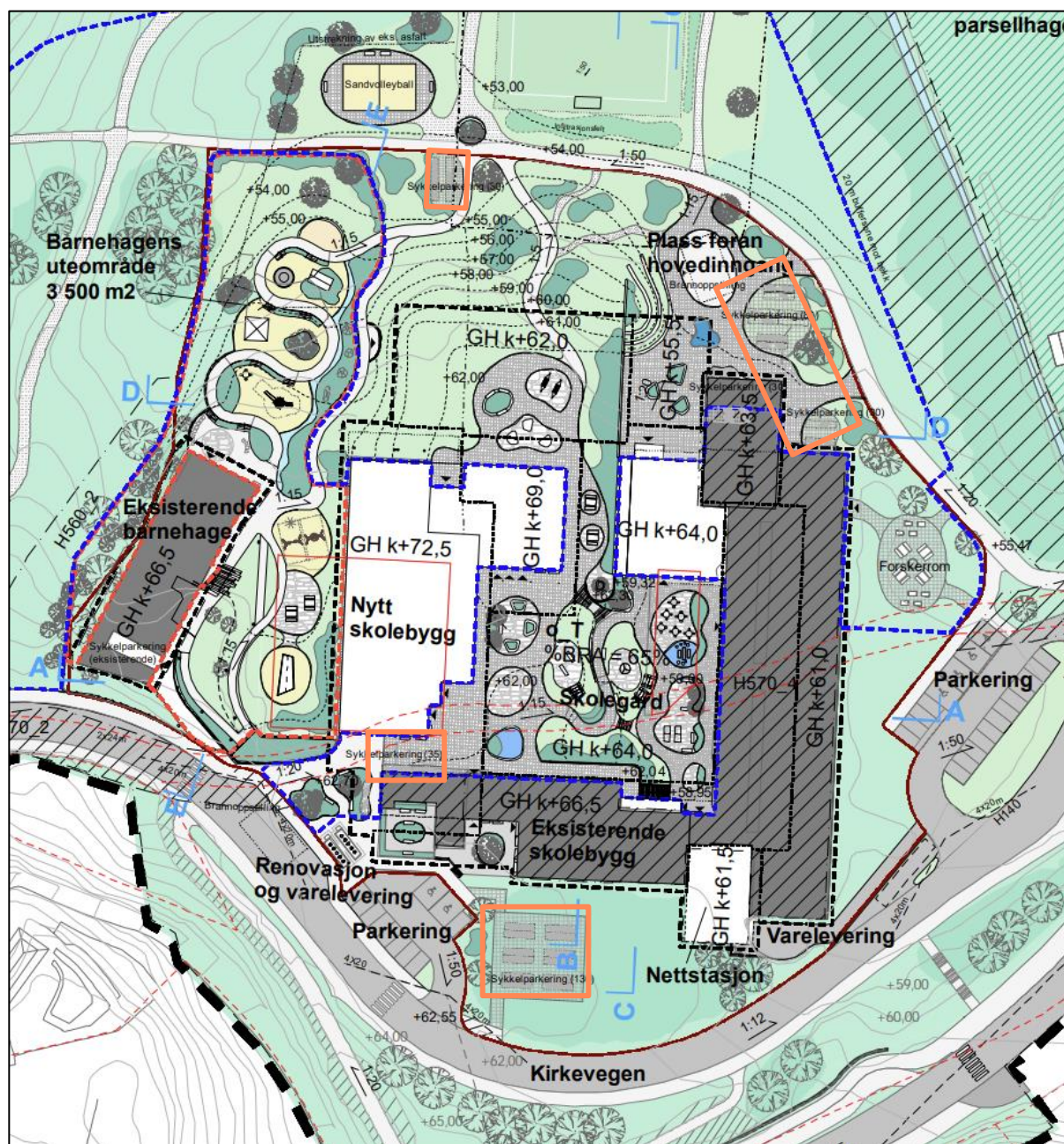
Figur 30 Mulig plassering av sykkelparkeringsplasser
