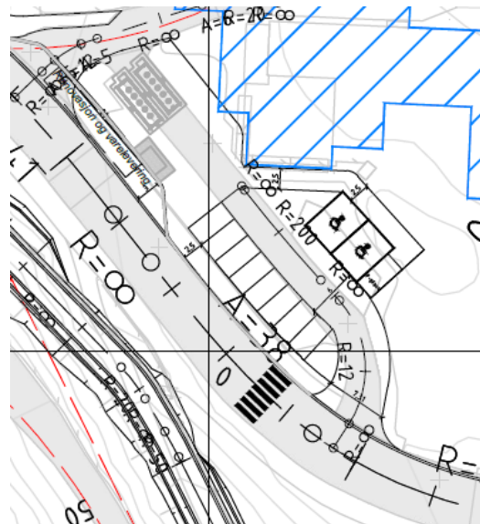
Figur 25 Ny gangfeltkryssing ved parkering i vest
