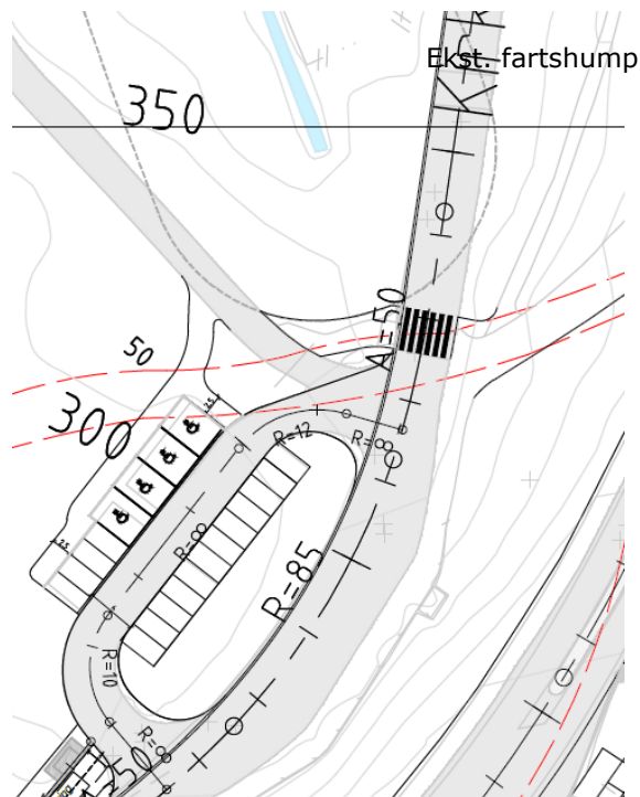
Figur 26 Utbedring av gangfelt i øst
