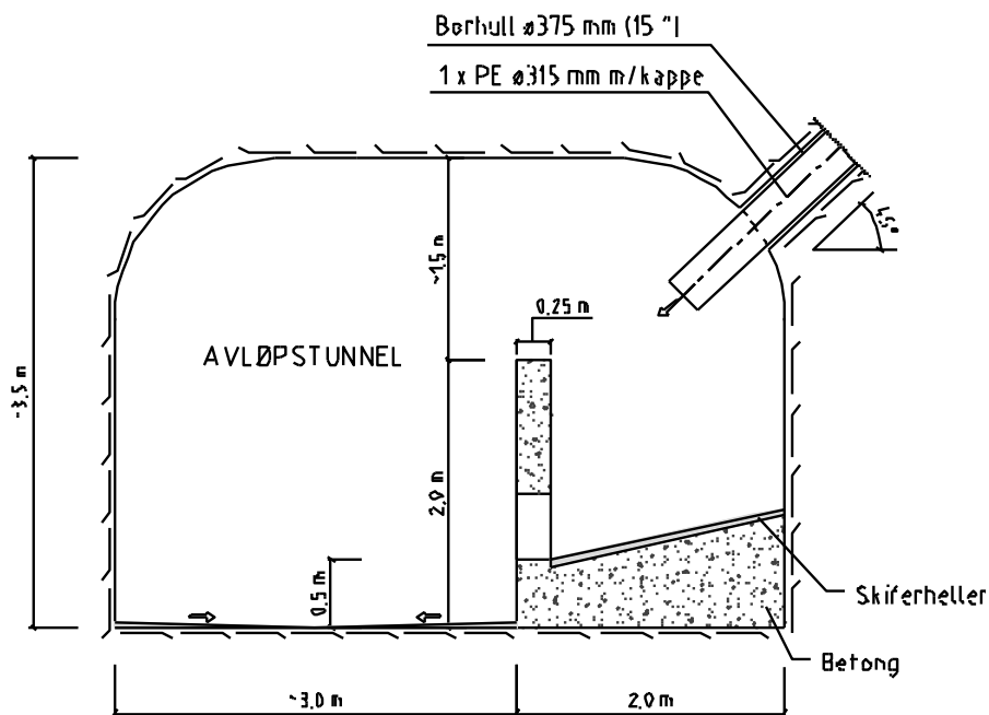
SNITT B-B
