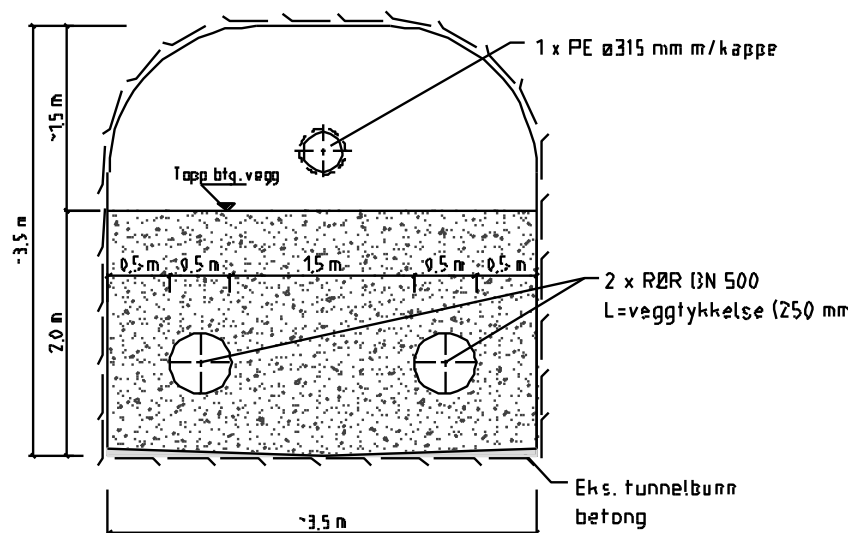
SNITT A-A
