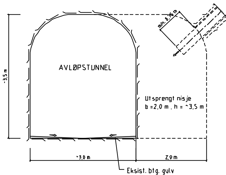
SNITT
