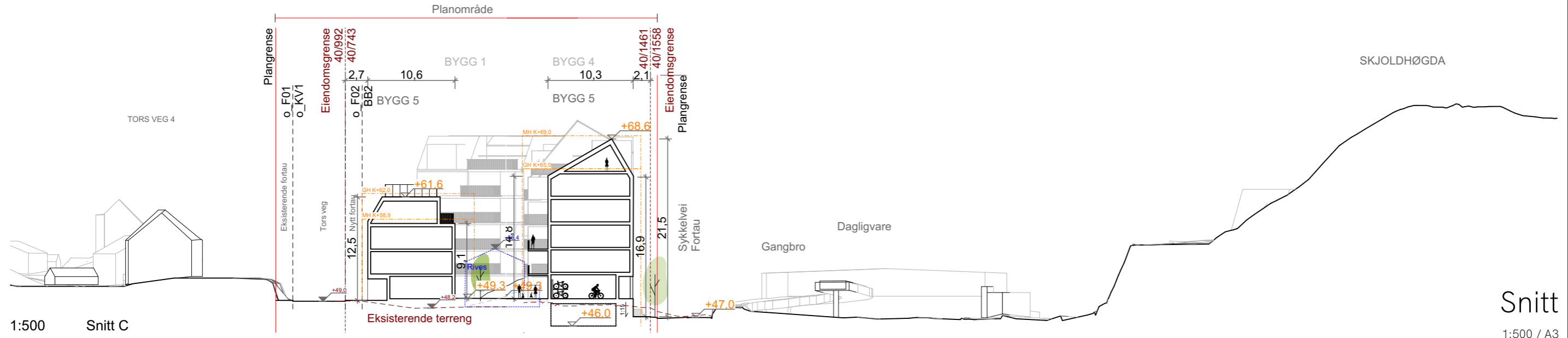
1:500 Terrengsnitt B
