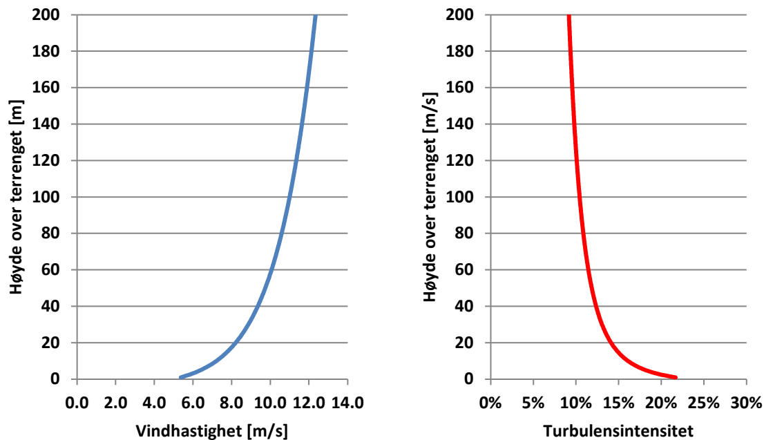
Figur 15: Grensebetingelser for hastighet og turbulens, her vist med en ruhet langs bakken som tilsvarer en implisitt modellering av nabobebyggelse. Profiler basert på ruhetslengden av vannoverflate er også brukt i analysen, men er ikke vist her. Referansehøyde for vindprofilene brukt i simuleringene er 58,0 m over terrenget/havet.
