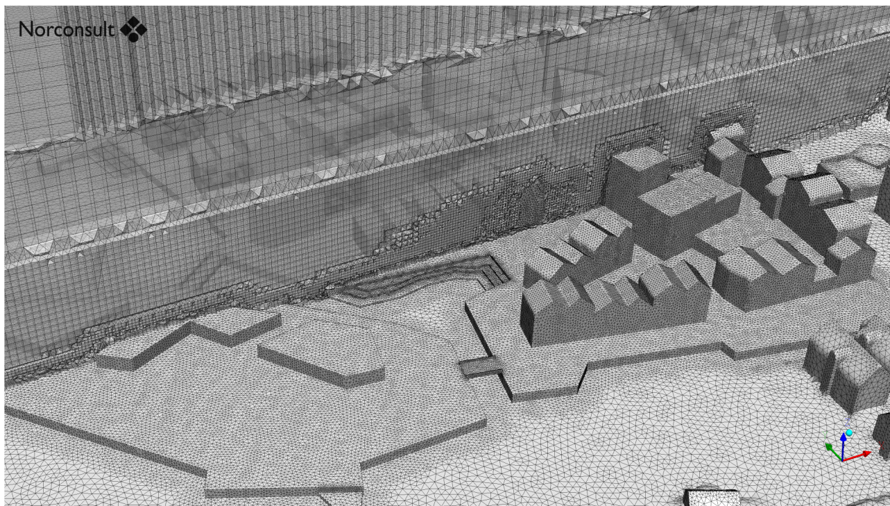
Figur 13: Visualisering av «meshet» langs overflater og et snitt gjennom volumet.
