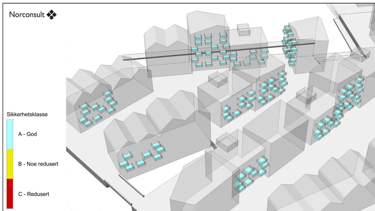
Figur 11: Sikkerhetskart i kroppshøyde for balkonger. Sett fra sørvest.
