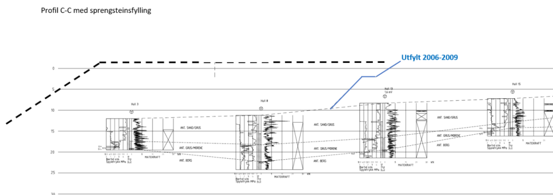
Figur 6-3: Skisse som viser profil C-C med sprengsteinsfylling med stabil skråningshelning.
