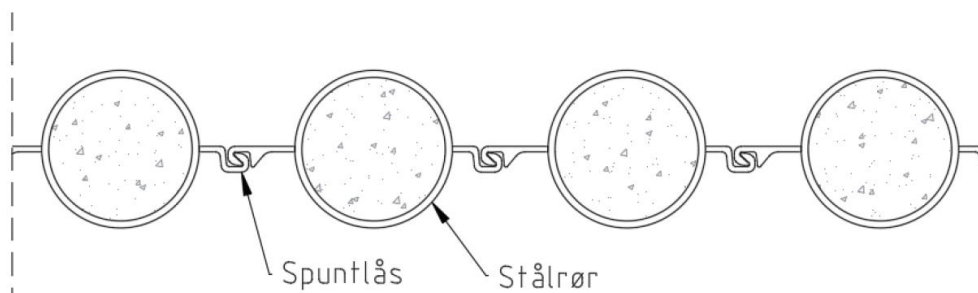
Figur 6-6: Prinsipskisse av rørspunt (kilde: Byggegropveilederen 2018).
