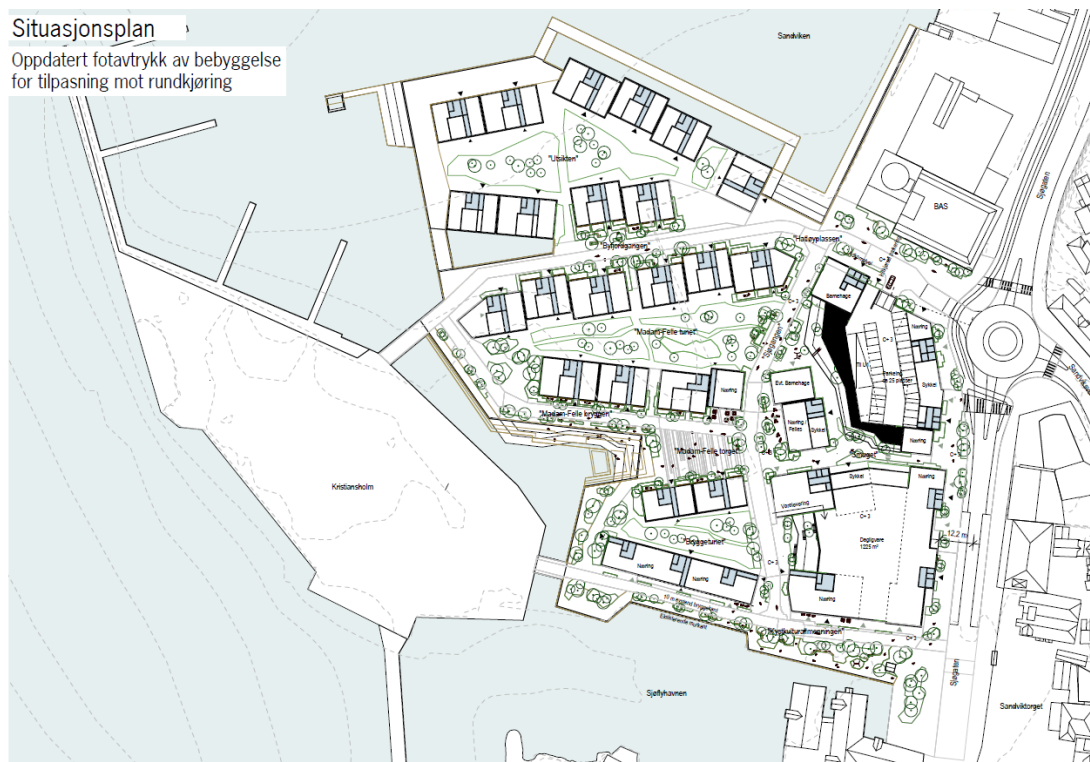
Figur 3 Plan for utbygging av området. Kristiansholm som holme re-etableres ved at det graves ut en kanal mellom boligområdet og planlagt friområde på holmen.
