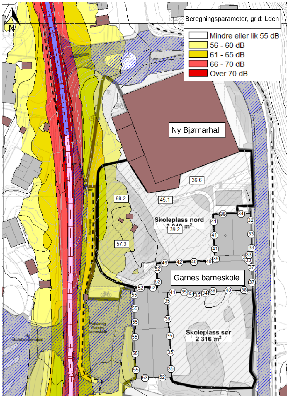
Figur 5 Støynivå, L_{den} (dB), på uteareal og ved fasade. Uskjærmet situasjon med ny idrettshall. Beregningshøyde er 1,5 m over terreng. Beregningspunkter ved fasade viser høyeste støynivå uavhengig av etasje. Skolens uteoppholdsareal er markert med tykk svart strek.
