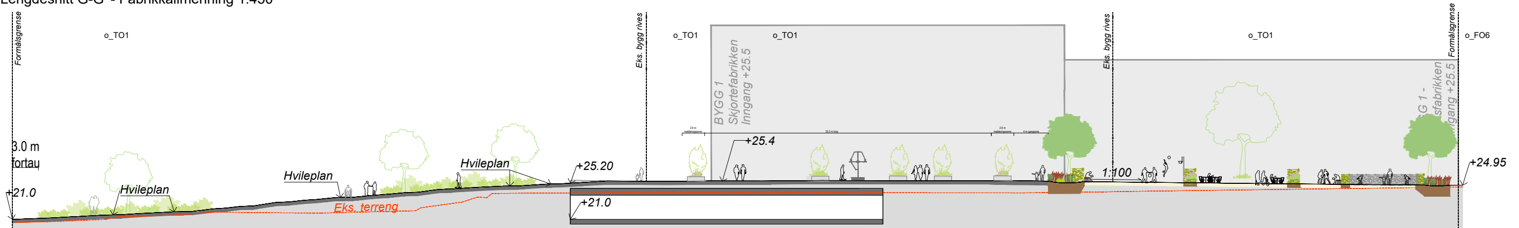
Lengdesnitt G-G' - Fabrikallmenning 1:450
