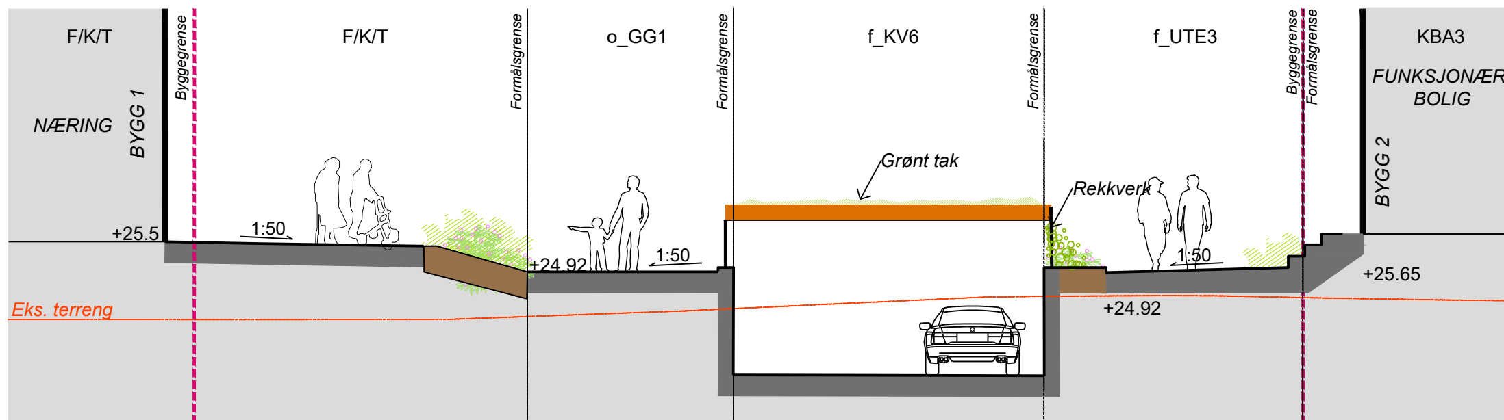
Prinsippsnitt K-K' 1:100
