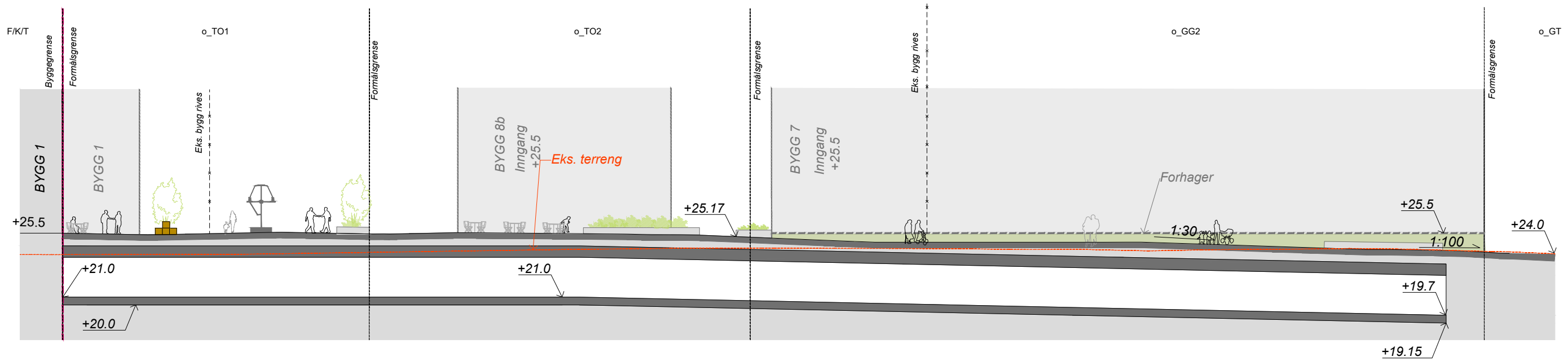
Lengdesnitt H-H' - Boliggaten 1:300
