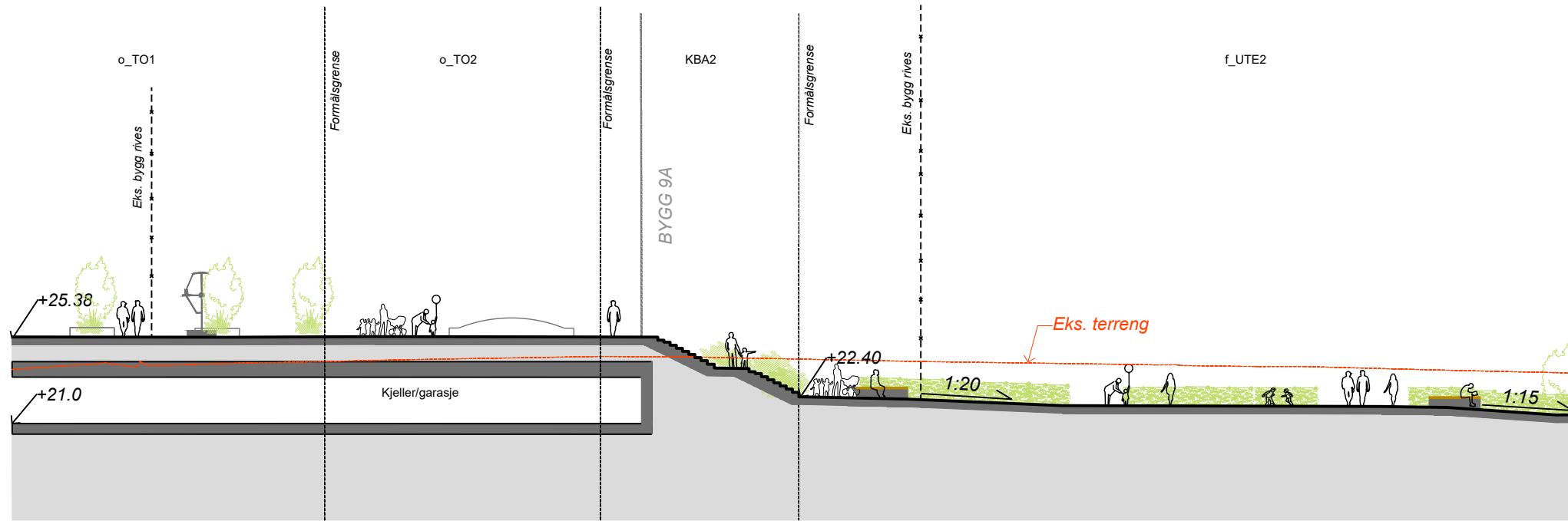
Lengdesnitt I-I' - Torg og Mindehagen 1:300
