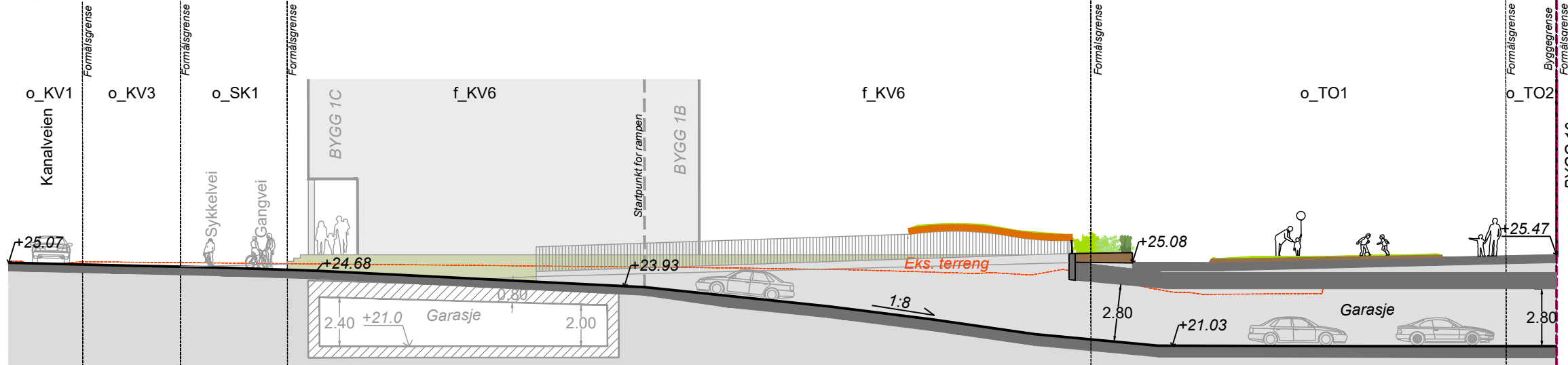
Lengdesnitt J-J' 1:250
