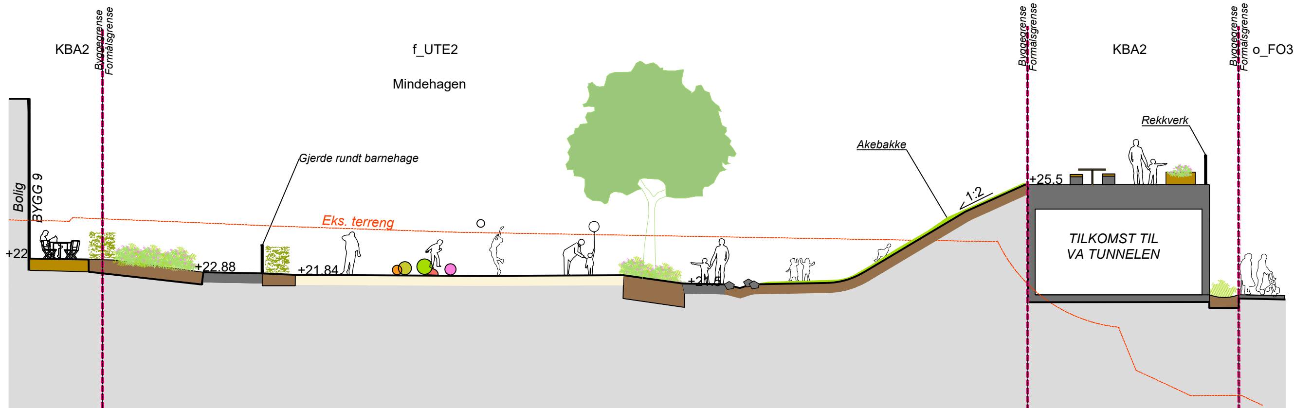
Prinsippsnitt Q-Q' 1:150
