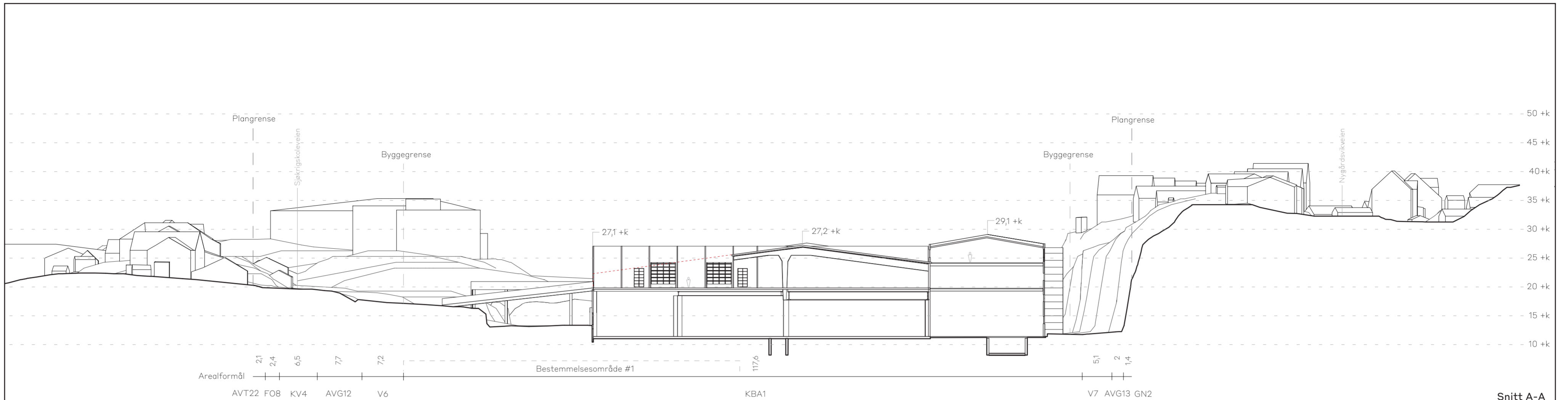
Snitt A-A
