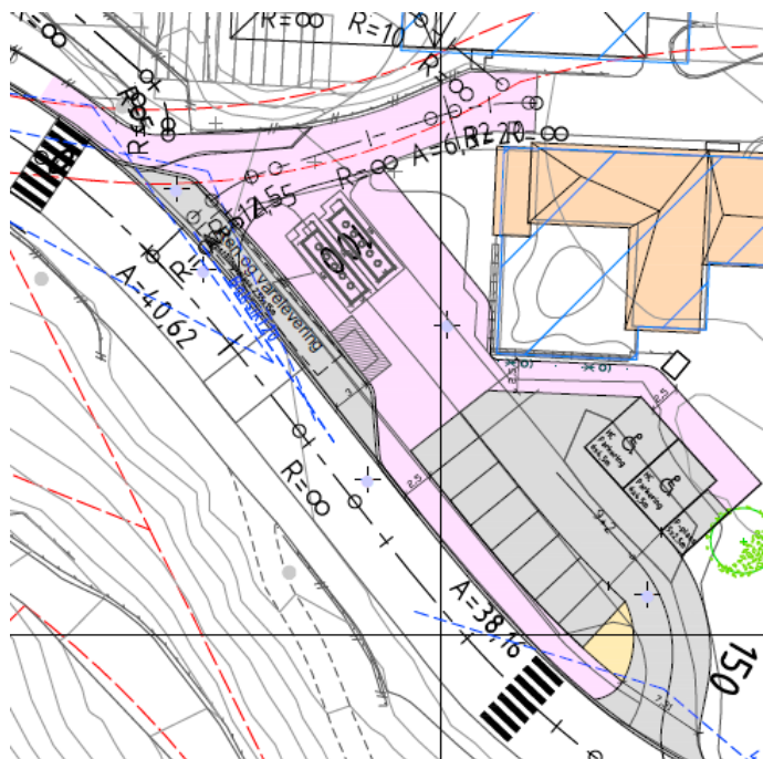
Figur 9 Lomme for renovasjon og varelevering ved barnehagen
