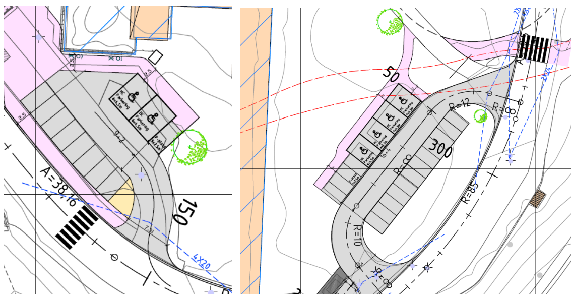
Figur 6 Bilparkering i vest og øst
