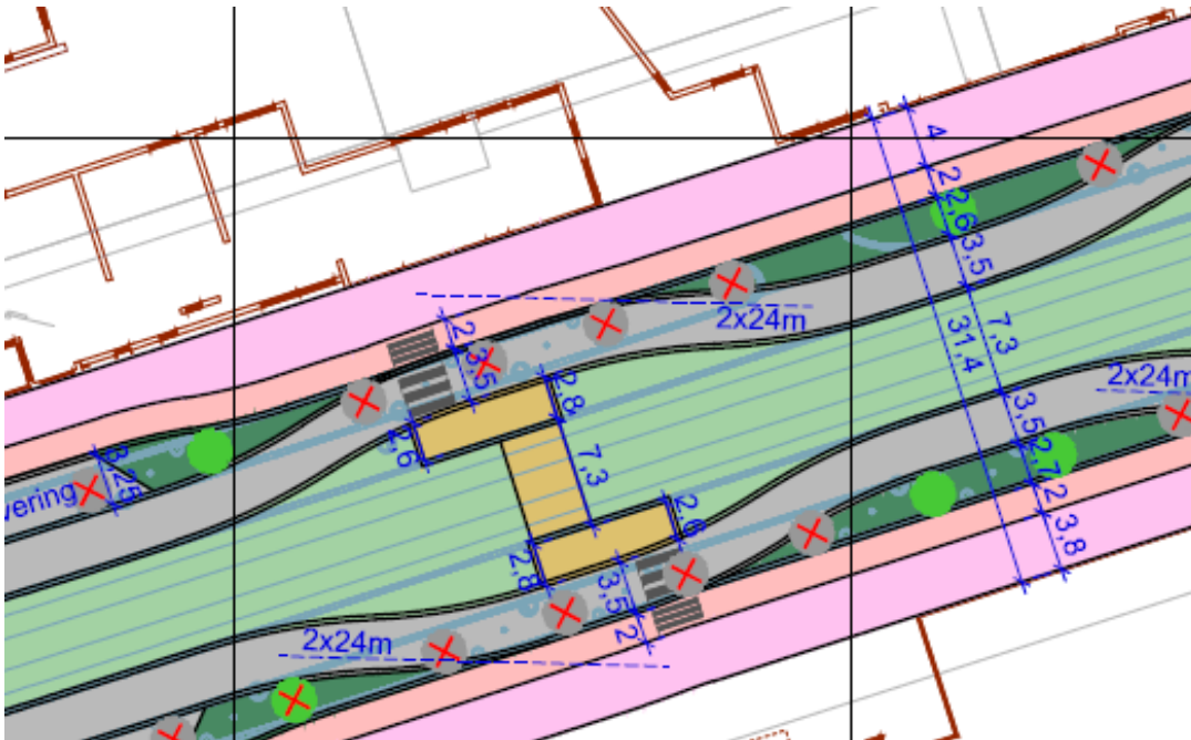
Figur 4-4 Skissen viser et av gangfeltene i alternativ 1A-b, med tilhørende bredder og mål.
