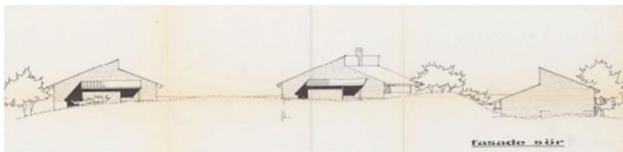
Figur 3: Teglsteinsbygningen ligger naturlig i terrenget, og hovedvolumene trapper seg ned mot øst. Tegningen viser fasaden mot sør. (Kilde: Byggesaksarkivet, Bergen kommune)
