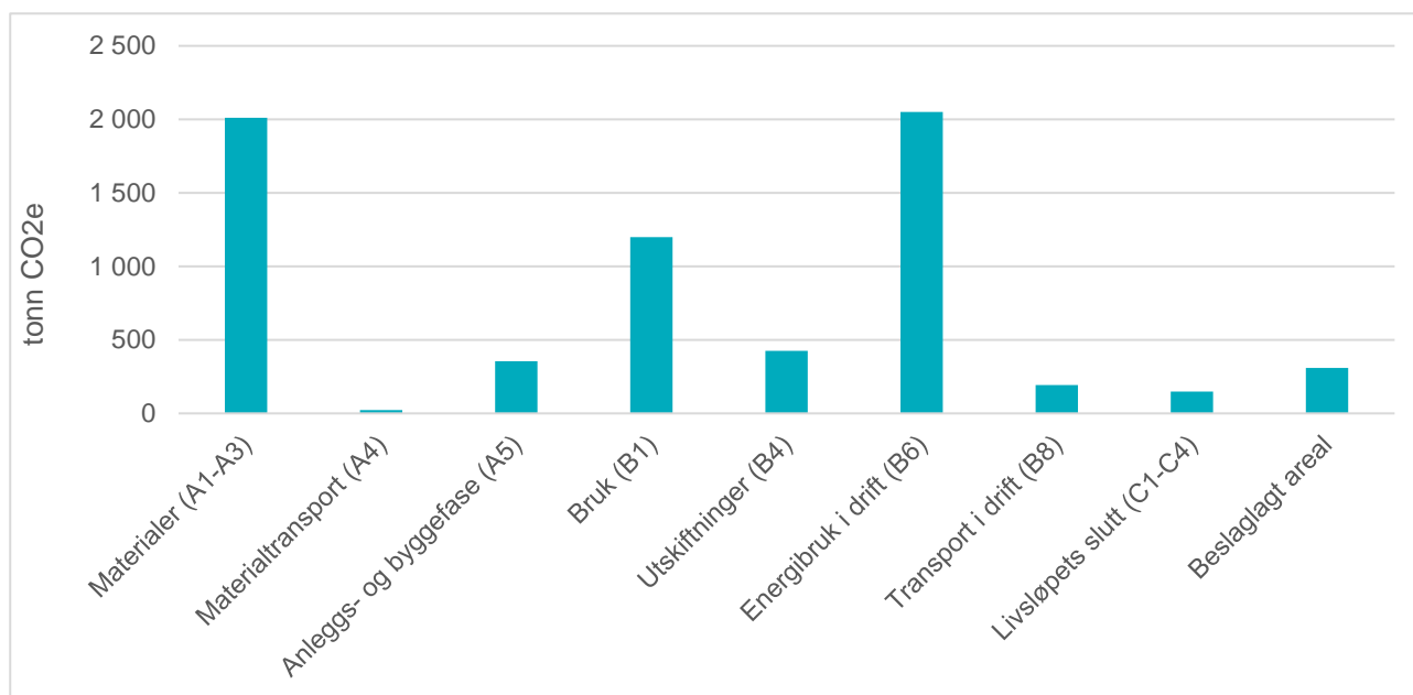
Figur 1: Beregnede klimagassutslipp vist i tonn CO 2 e per livsløpsfase.
