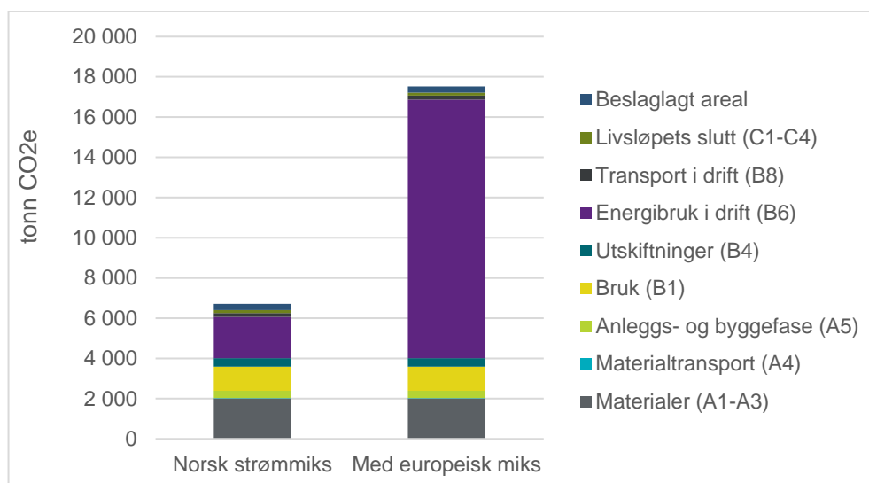
Figur 3: Klimagassutslipp fordelt på livsløpsfaser, vist ved bruk norsk og europeisk strømmiks i tonn CO 2 e.
