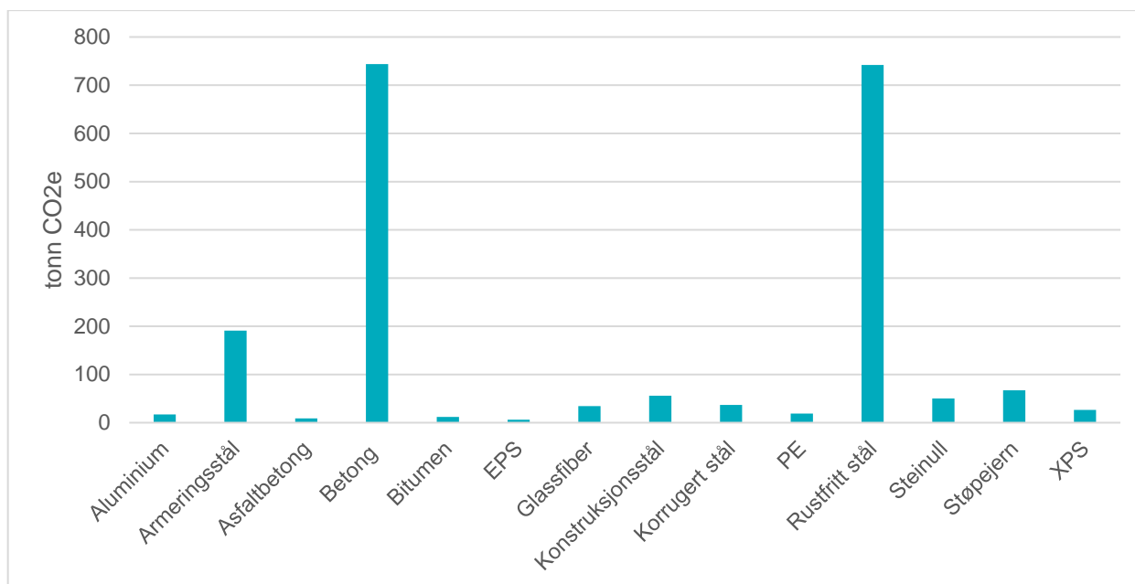
Figur 2: Beregnede klimagassutslipp vist i tonn CO 2 per materiale for livsløpsfase A1 – A3.
